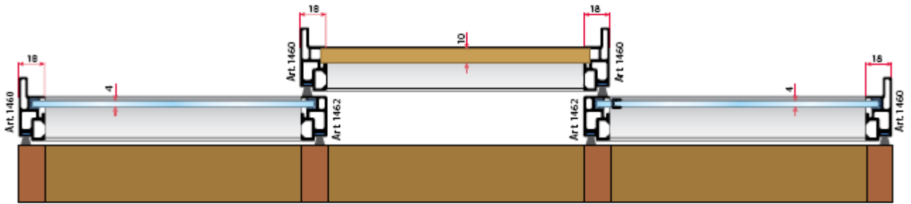
Вариант трехдверного шкафа - вид сверху
